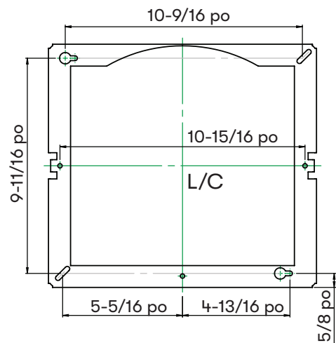
CADRE de FIXATION SUPÉRIEUR
