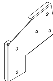
A4M00512 | EXTENSION DE POUTRE (1) | DE BALANÇOIRE SUPPORT BLEU - DROIT
