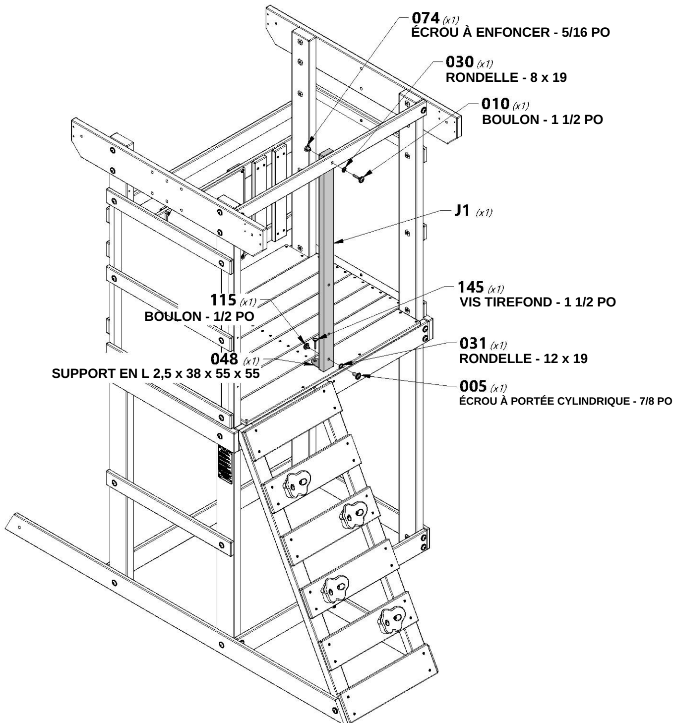
H100030 | RONDELLE DE (1) | VERROUILLAGE EXT 8 x 19
