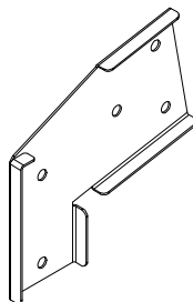
A4M00511 | EXTENSION DE POUTRE (1) | DE BALANÇOIRE SUPPORT BLEU - GAUCHE
