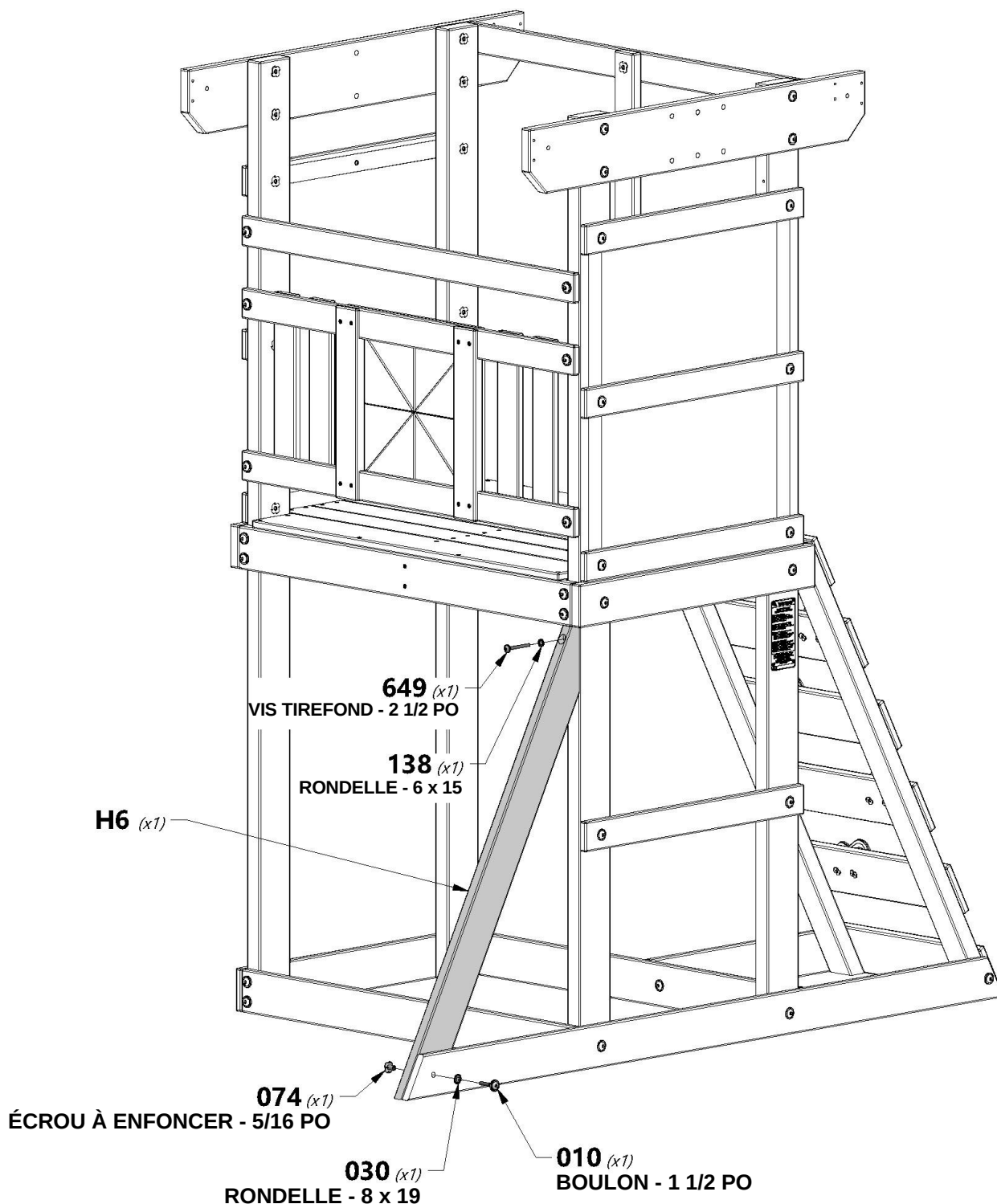
H100030 | RONDELLE DE VERROUILLAGE EXT (1) 8 x 19
