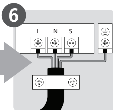
6 Raccordement du câblage (Page 15)
