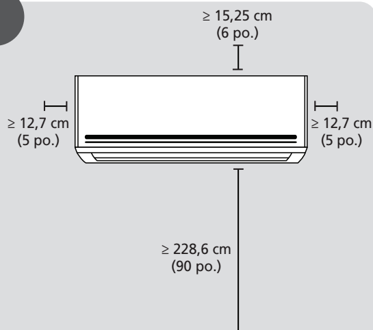
Choix du lieu d'installation (Page 9)
