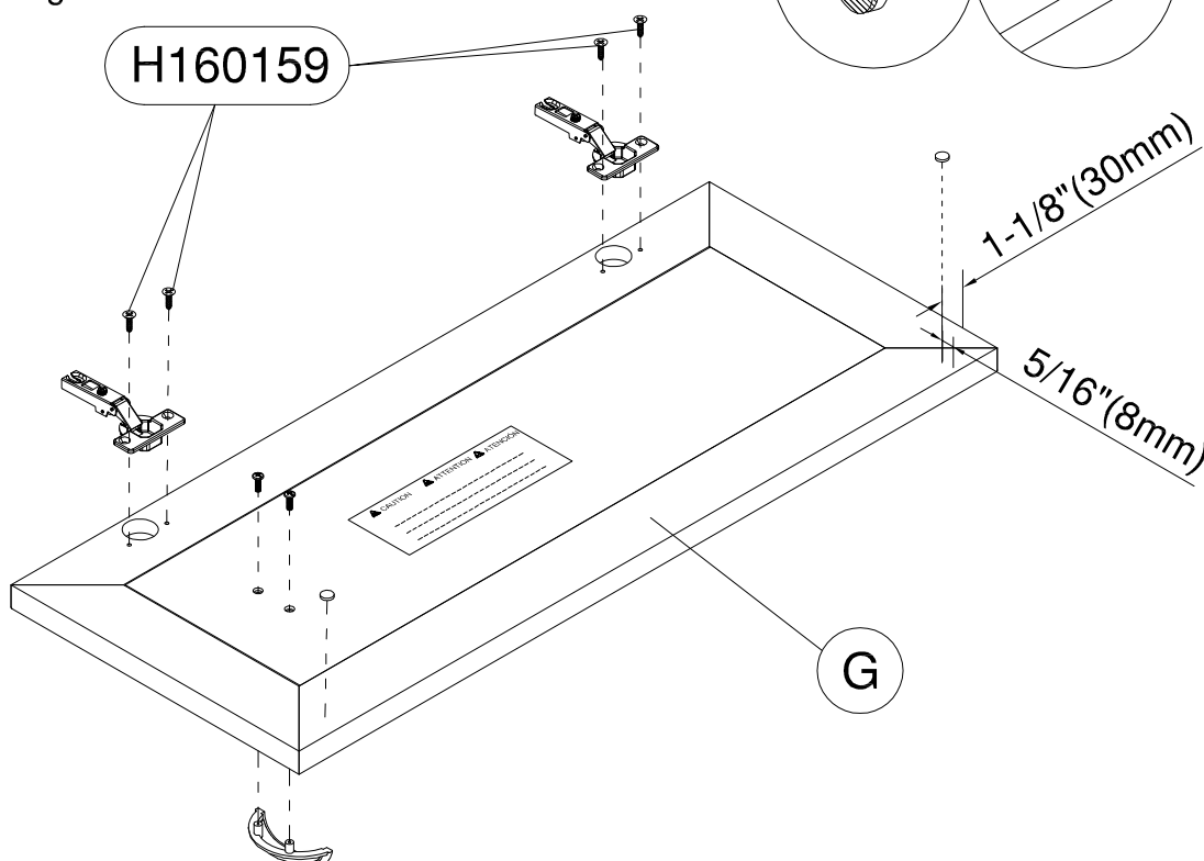
Hinge
