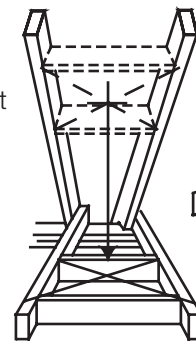
Espaceur coupe-feu face inférieure des solives
