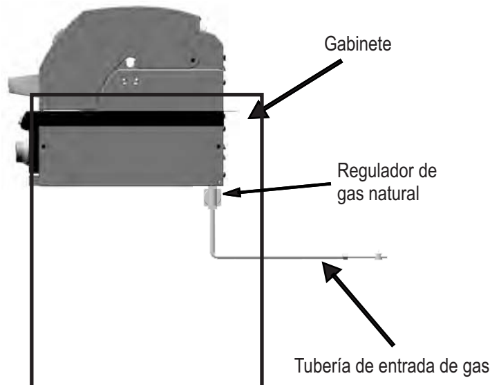
Figura 7 Vista lateral
