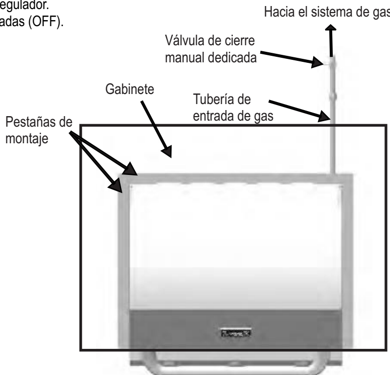
Figura 8 Vista superior
