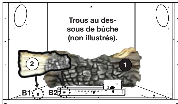
2. Placez les trous dans bûche n° 2 sur B1 et B2. Ne couvrez pas les orifices de brûleur.
