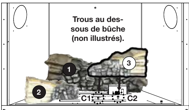
3. Placez les trous dans bûche n° 3 sur C1 et C2. Ne couvrez pas les orifices de brûleur.
