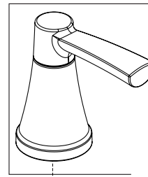
RP101879▲ Handle Assemblies Conjunto de manija Montage de la manette
