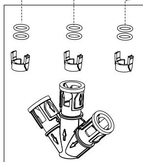
RP101296 Blocks & O-Rings Bloques y Aros-O Blocs de fixation et joints toriques
