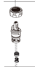
RP101504 Stem Unit Assembly, Seat & Spring, Bonnet Nut & Washer Ensamble de la Unidad del Vástago, Asiento y Resorte, Bonete y Arandela Obturbador, siège et ressort, écrou à chapeau et rondelle
