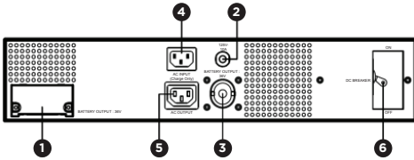
Back Panel: BP36VL2U01TAA
