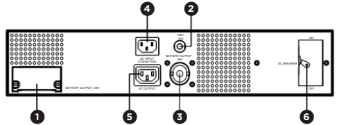
Back Panel: BP48VL2U01TAA
