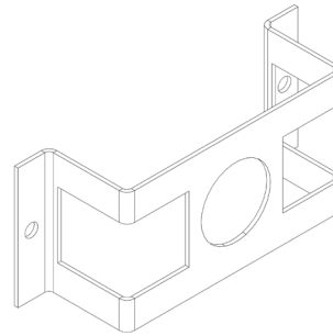
FIGURE 2 - SUPPORT POUR LE PURGEUR EXTERNE
