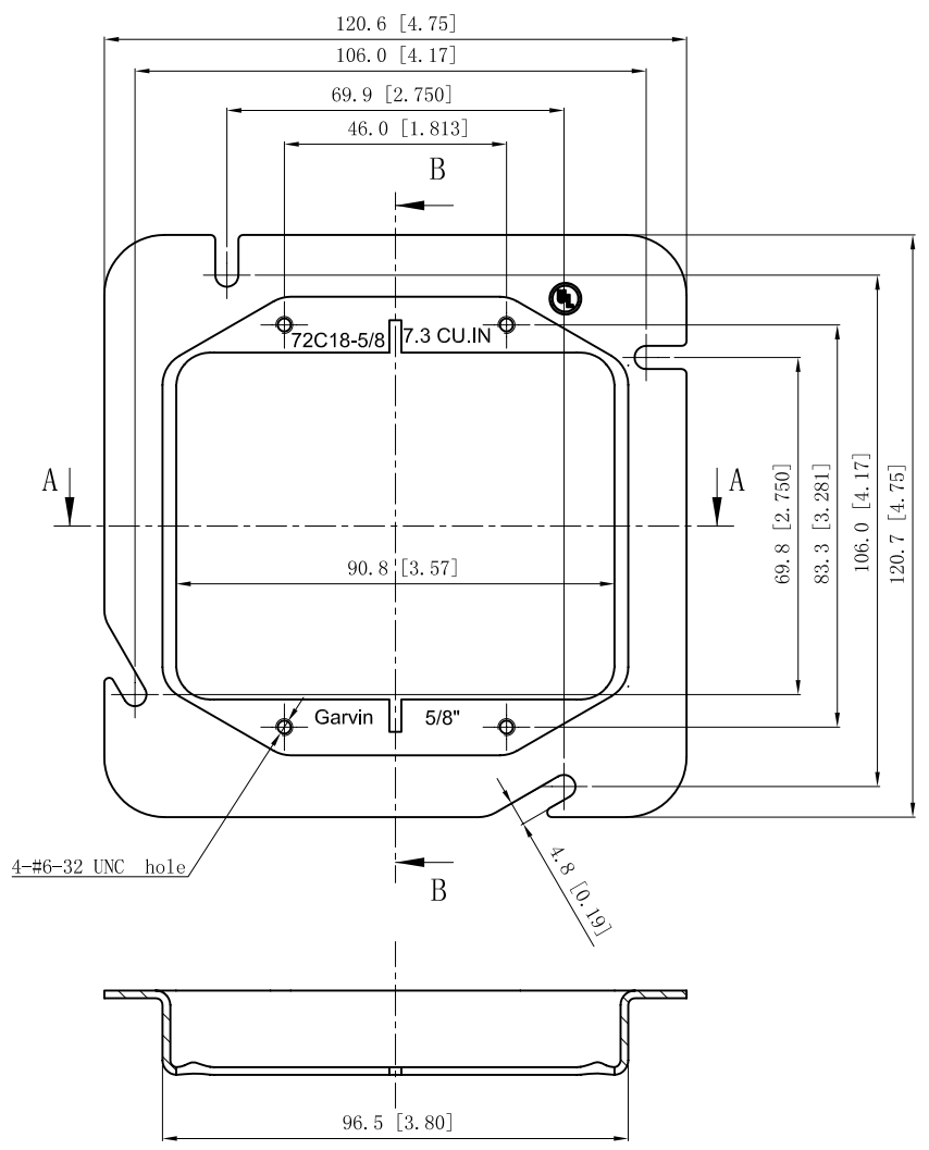
VIEW A-A
