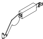
x2 RP413184-HINGEL Left Safety Lift Hinge* Support de couvercle (gauche) Soporte tapa (izquierda)
