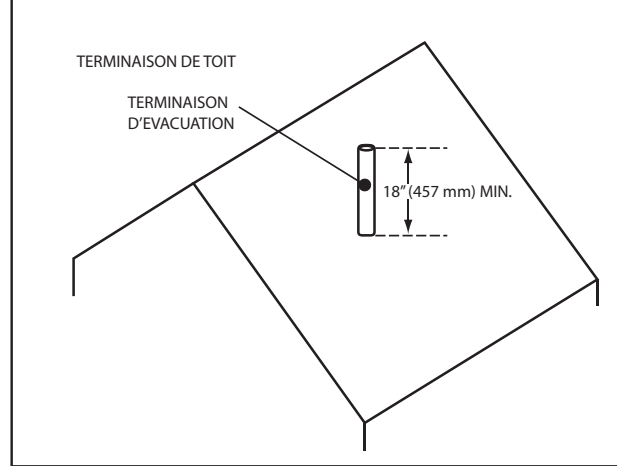
FIGURE 10 - ÉVACUATION VERTICALE
