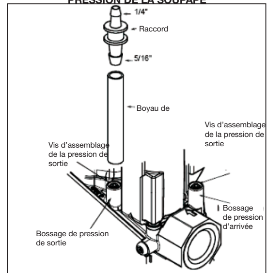
FIGURE 29 - ENSEMBLE DE VÉRIFICATION DE LA PRESSION DE LA SOUPE
