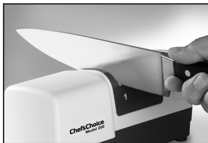
Figura 1. Inserimento della lama nell'alloggiamento sinistro della fase 1. Alternare singoli passaggi nell'alloggiamento destro e sinistro.
