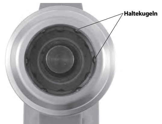
Abbildung 8 – Das Innere der QCS-Kupplung
