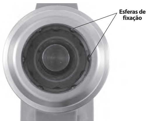
Figura 8 – Interior de um acoplamento QCS
