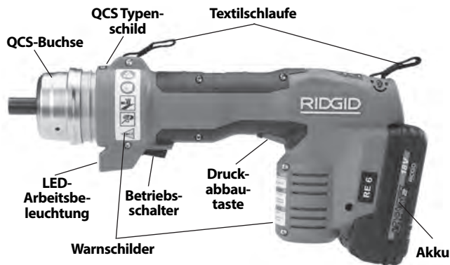
Abbildung 1 – RE 6/RE 60 - QCS-Kupplung zum Anbringen des Kopfes verwenden
