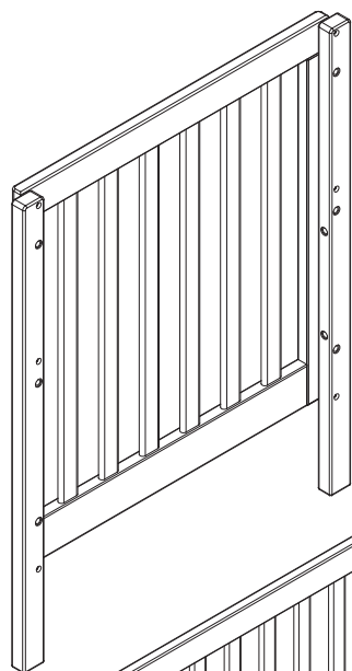
A. Crib End x 2 Extrémité du lit pour bébé x 2 Extremo de la cuna x 2 27849
