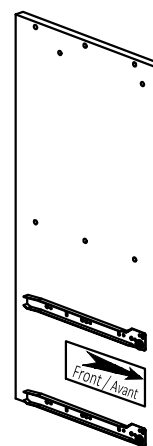
RIGHT DIVIDER QTY 1
