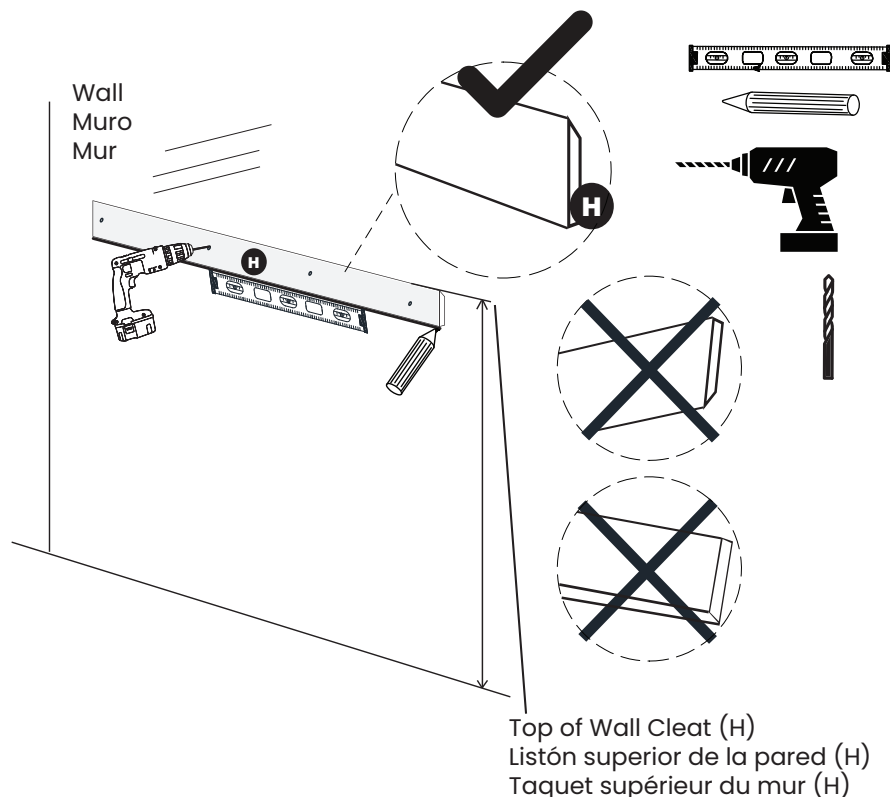
Bottom height of locker Altura inferior del casillero Hauteur inférieure du casier
