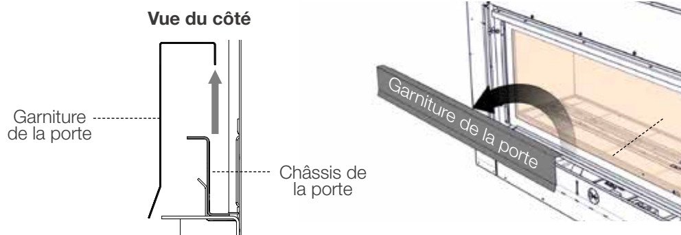
TLV50 Illustrée
