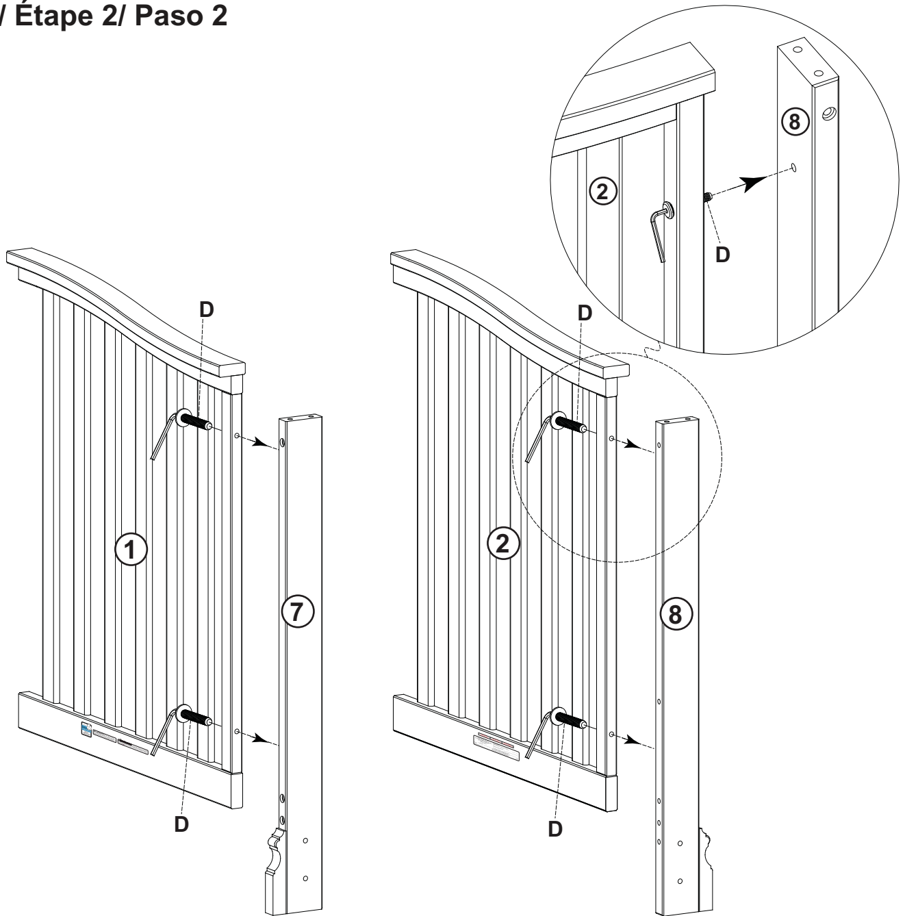
Left Front Post Montant avant gauche Poste frontal izquierdo
