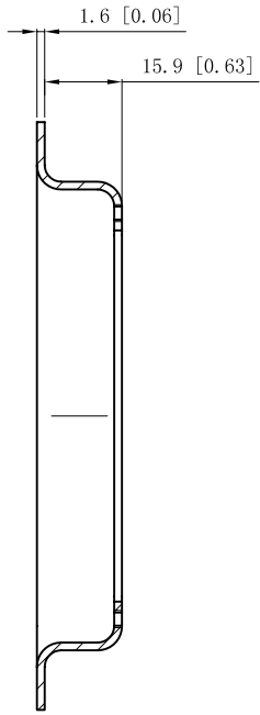
VIEW A-A
