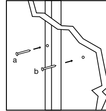
Verwenden Sie eine Flachkopfschraube (Nr. 10) für Wände mit Ständerprofil. a) Verwenden Sie Dübel (Nr. 10) und Schrauben ausreichender Stärke für Wände ohne Ständerprofil. b) Lassen Sie die Schrauben etwa 4 mm herausstehen.
