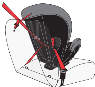
Ceinture sous-abdominale et baudrier
