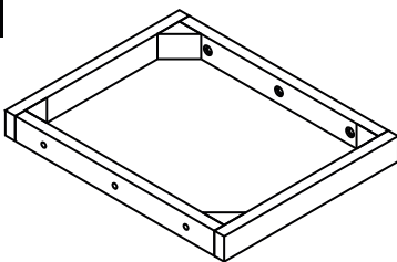
BOTTOM FRAME QTY 1
