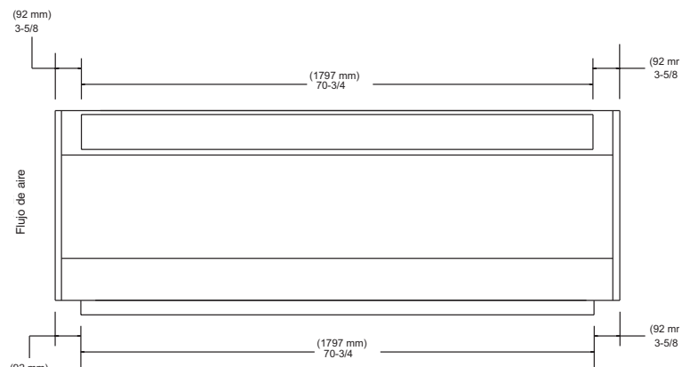
VISTA FRONTAL GABINETE DE 1981 mm (78 PULG.)
