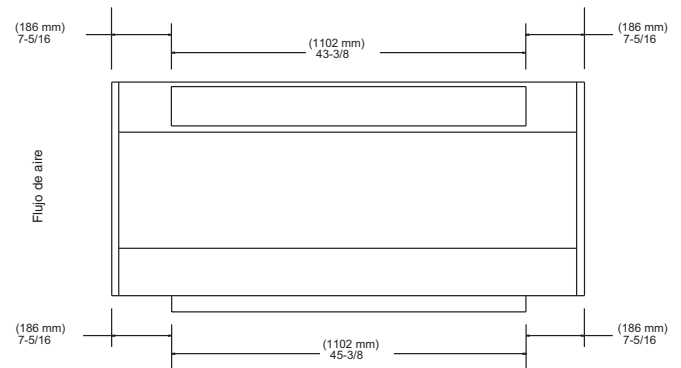
VISTA FRONTAL GABINETE DE 1473 mm (58 PULG.)
