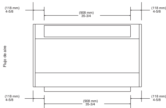
VISTA FRONTAL GABINETE DE 1143 mm (45 PULG.)
