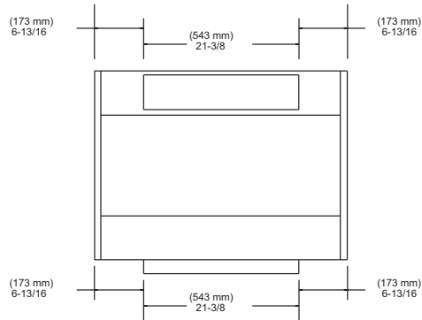
VISTA FRONTAL GABINETE DE 889 mm (35 PULG.)
