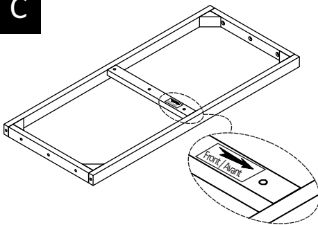
BOTTOM SHELF QTY 1
