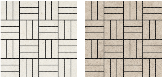
Alcor Orion
