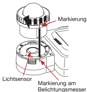
Lumisphere-Verriegelung 1
