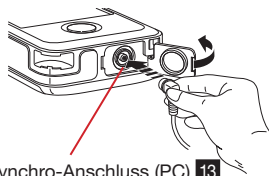
Synchro-Anschluss (PC) 13
