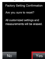
Bestätigungsbildschirm
