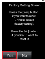
Bestätigungsbildschirm
