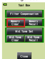
Werkzeugbildschirm
