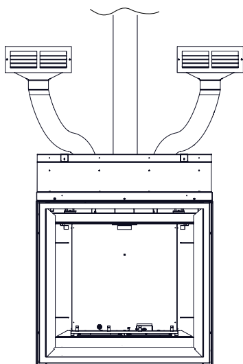
Sortie arrière / supérieure
