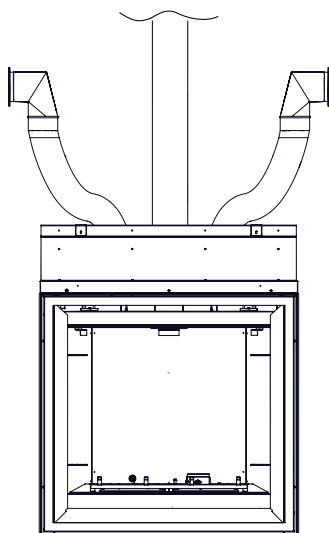
Sortie arrière / supérieure
