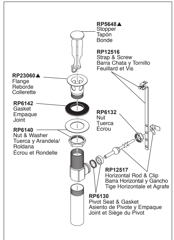
RP26533▲ Metal Pop-Up Assembly Less Lift Rod Ensemble de Metal del Desagüe Automático Menos la Barra de Alzar Renvoi Mécanique en Métal Sans la Tige de Manoeuvre
