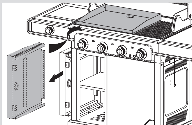
Colocación correcta de la placa plancha
