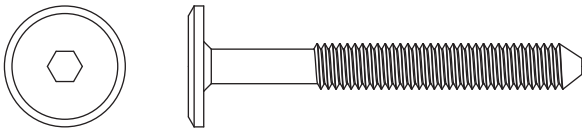
C. M6x50 mm Φ17 Head Bolt x 1 Boulon à tête hexagonale Φ17 M6x50 mm x 1 Perno de Cabeza Φ17 M6x50 mm x 1 5981
