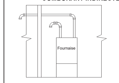
FIGURE 7 - PRISE D'AIR COMBURANT INDIRECTE
