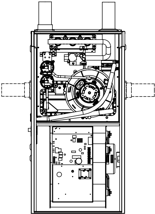
ÉVENT SUPÉRIEUR - DRAIN À GAUCHE INSTALLATION (INTERNE)
