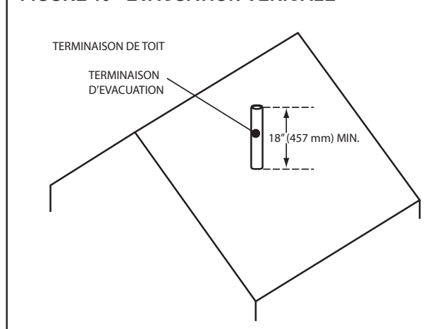
FIGURE 10 - ÉVACUATION VERTICALE
