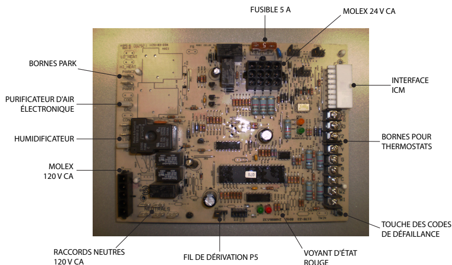
FIGURE 32A - CONTRÔLE D'ALLUMAGE DE FOURNAIE INTÉGRÉ
