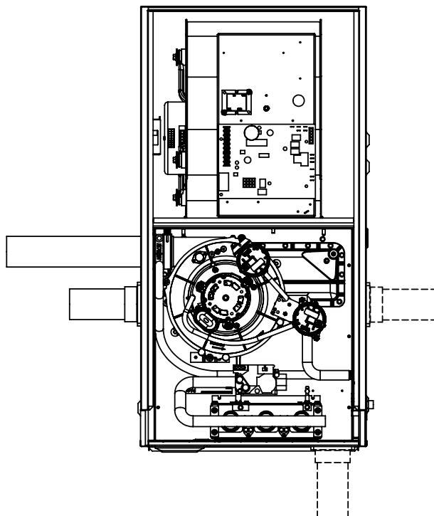
FIGURE 19 - OPTION D'ÉVACUATION ET DE DRAINAGE VERS LE BAS
