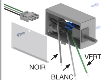
FIGURE 31 - BRANCHEMENTS ÉLECTRIQUES/ CONNECTEUR MOLEX
