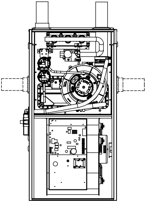
ÉVENT SUPÉRIEUR - DRAIN À GAUCHE INSTALLATION (EXTÉRIEUR)
