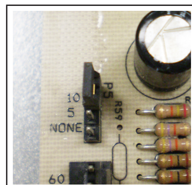
FIGURE 32 - FIL DE DÉRIVATION P5
