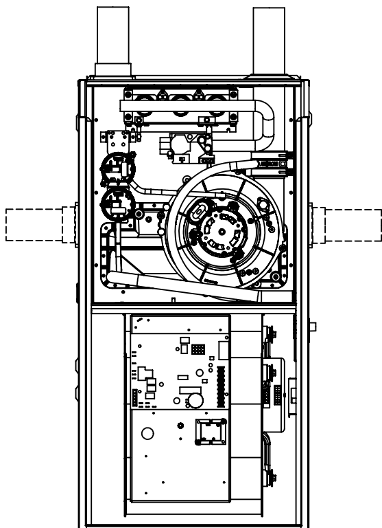
FIGURE 16 - OPTION D'ÉVACUATION ET DE COURANTE ASCENDANTE (CONTINU)
