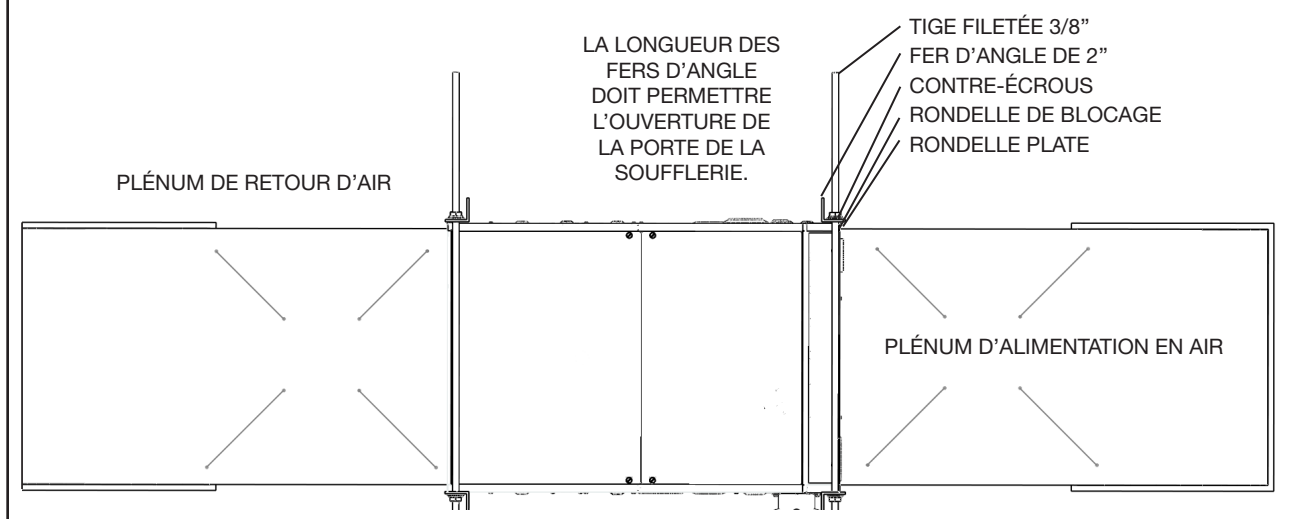
FIGURE 3 - MÉTHODE SUGGÉRÉE DE SUSPENDRE LA FOURNAISE HORIZONTALE
