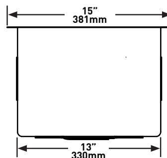
Vista lateral de la sección transversal
