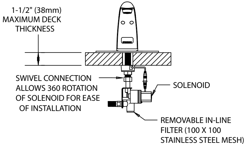
S-8710-CA-E S-8711-CA-E
