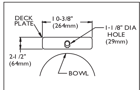
S-8720-CA-E S-8721-CA-E
