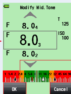
Écran « Modify Current Mid. Tone » (Modifier Mid. Tone actuel)
