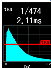
Écran « Flash Duration Analysis Cordless Mode Flash Waveform Graph » (Graphique de la puissance du flash en mode Analyse de durée du flash sans fil)
