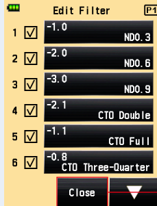
Écran « Edit Filter » (Modifier le filtre)
