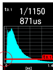
Mode flash sans fil
