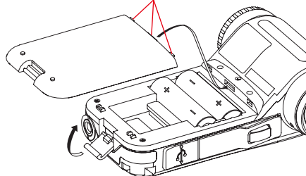
Compartiment des Piles 20
