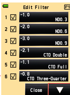
Edit Filter (Modifier le filtre) Page 1
