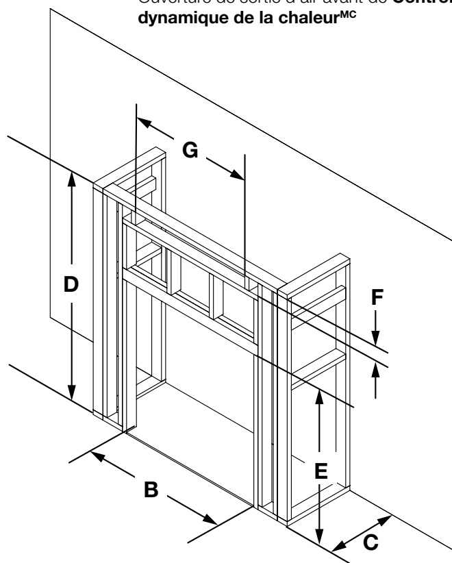
Option d'Installation 2 illustré
