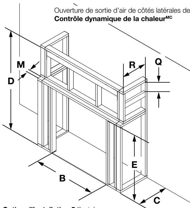
Option d'Installation 5 illustré
