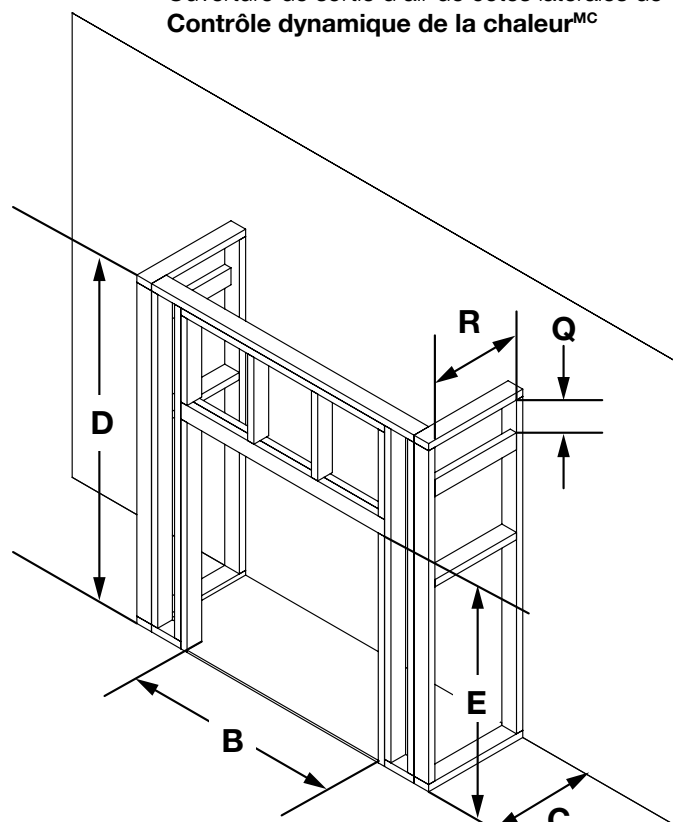
Option d'Installation 5 illustré
