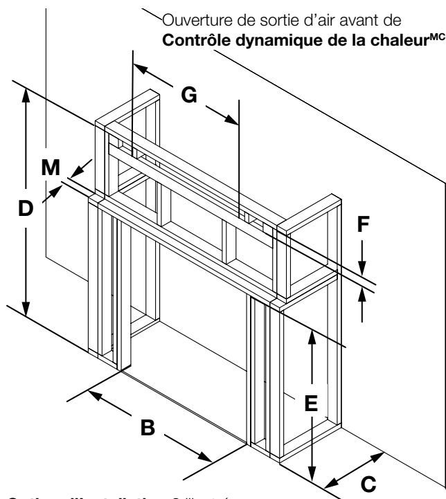
Option d'Installation 2 illustré
