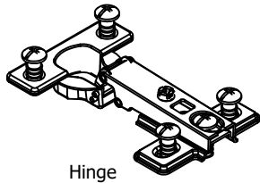
Hinge
