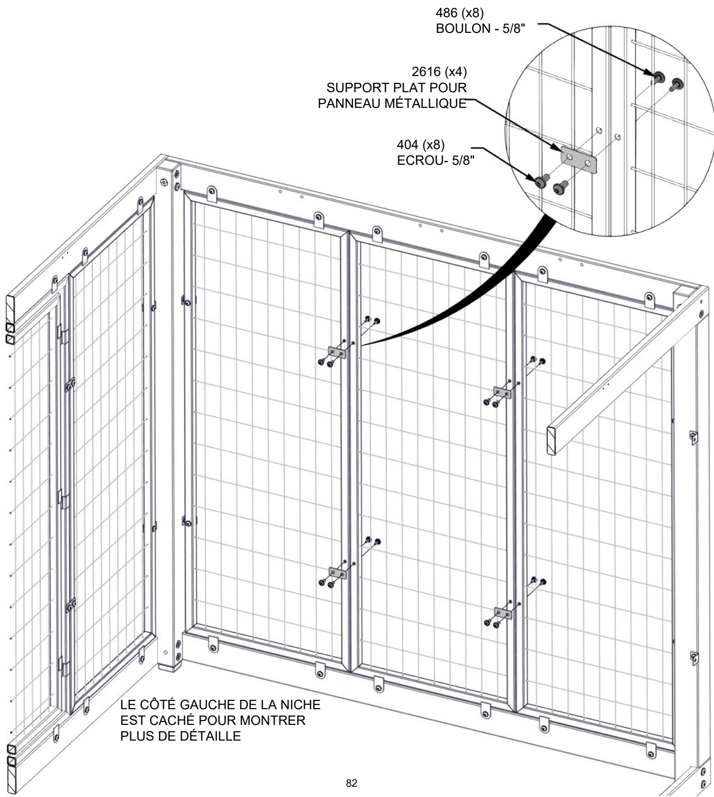
A4M02616 SUPPORT PLAT POUR PANNEAU MÉTALLIQUE (x4)
