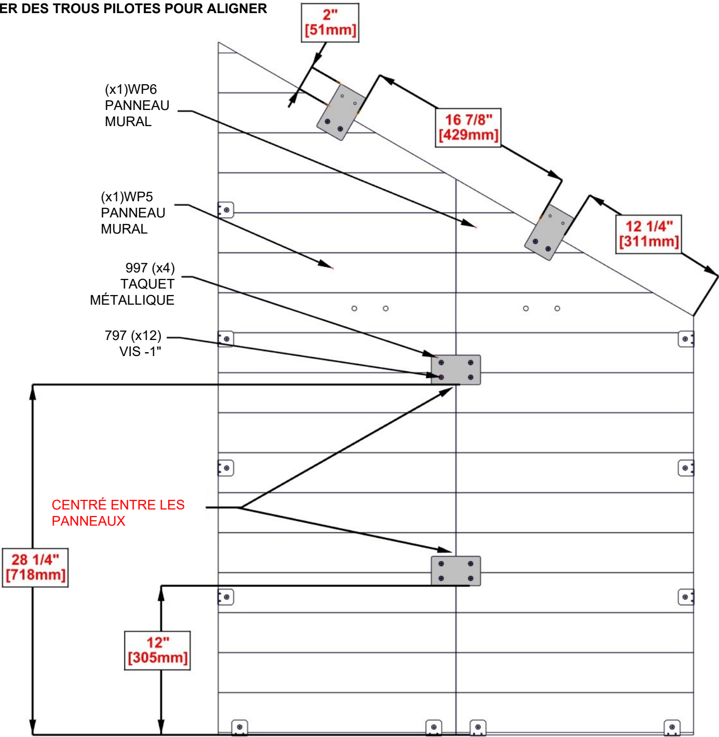
ENSEMBLE WP6 (x1) (DE L'ÉTAPE 18 A)
