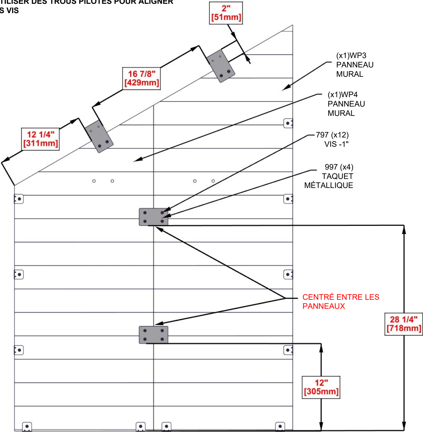
WP4 ENSEMBLE (x1) (DE L'ÉTAPE 19 A)
