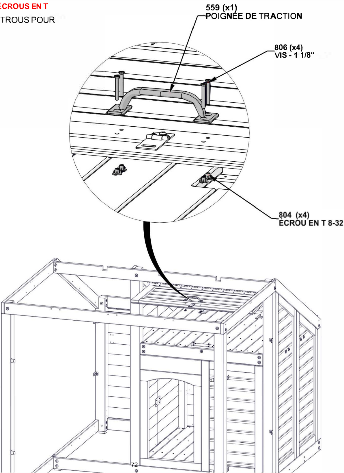
A4M00559 POIGNÉE DE TRACTION (x1)
