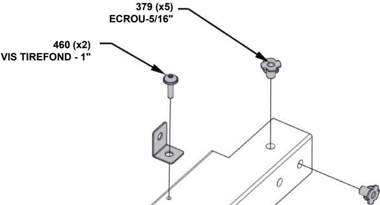
A4M02615 PIED DE POTEAU 2x2 (x2)
