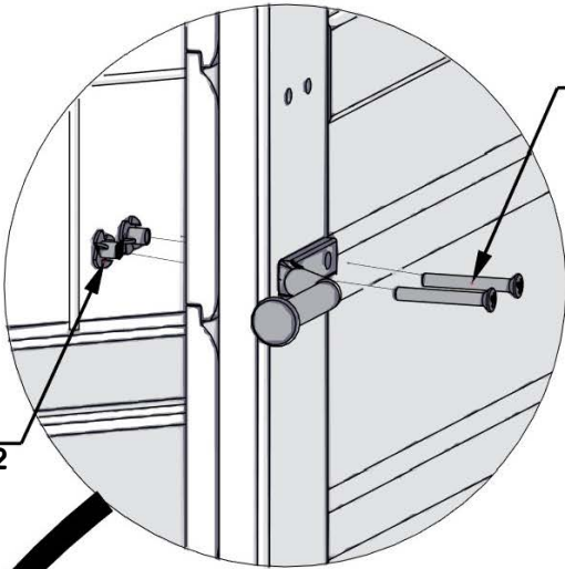
804 (x4) ÉCROU 8-32
