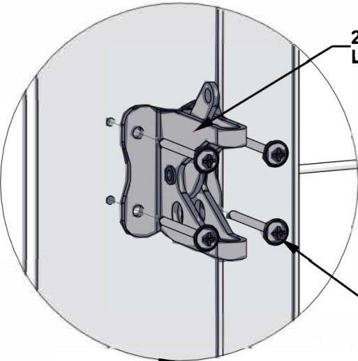
797 (x8) VIS - 1"
