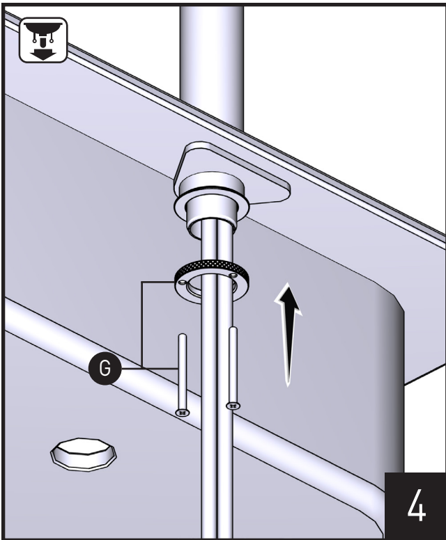
Install Mounting Nut [G] onto Mounting Shank. Installer l'écrou de montage [G] sur la tige de montage. Instale la tuerca de montaje [G] en la varilla de montaje.
