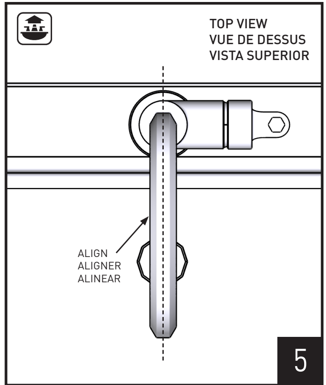
Check overall faucet alignment with sink drain hole from the top view. Vérifier, vu du dessus, l'alignement général du robinet sur l'orifice du drain du lavabo. Verifique la alineación general de la llave con el orificio de drenaje del lavabo desde la vista superior.
