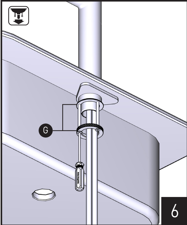
Tighten Mounting Nut [G] with screwdriver, once faucet alignment is confirmed. Une fois confirmé le bon alignement du robinet, serrer l'écrou de montage [G] avec le tournevis phillips. Apriete la tuerca de montaje [G] con la tournevis phillips, una vez que se confirme la alineación de la llave.
