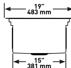
Vista lateral de la sección transversal
