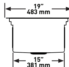
Coupe transversale - Vue latérale
