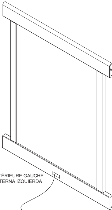
C. Left Post x 2 Poste gauche x 2 Poste Izquierdo x 2 26882
