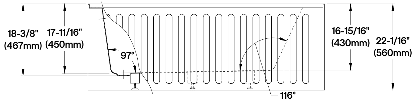
Section A-A
