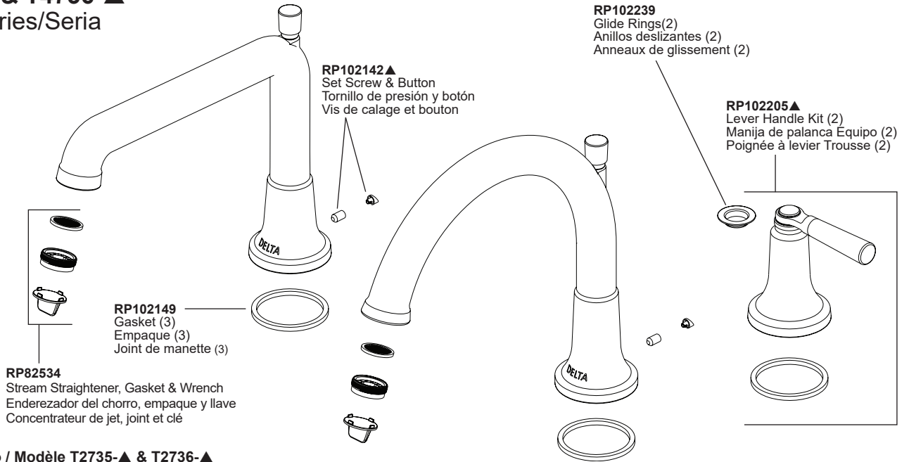
Model / Modelo / Modèle T2735-▲ & T2736-▲
