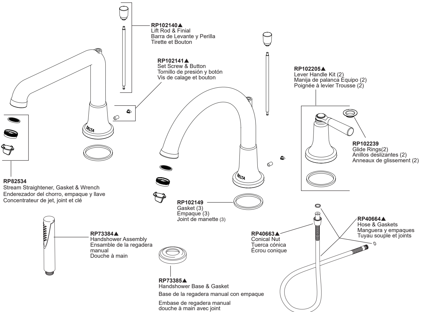
Model / Modelo / Modèle T4735-▲ & T4736-▲
