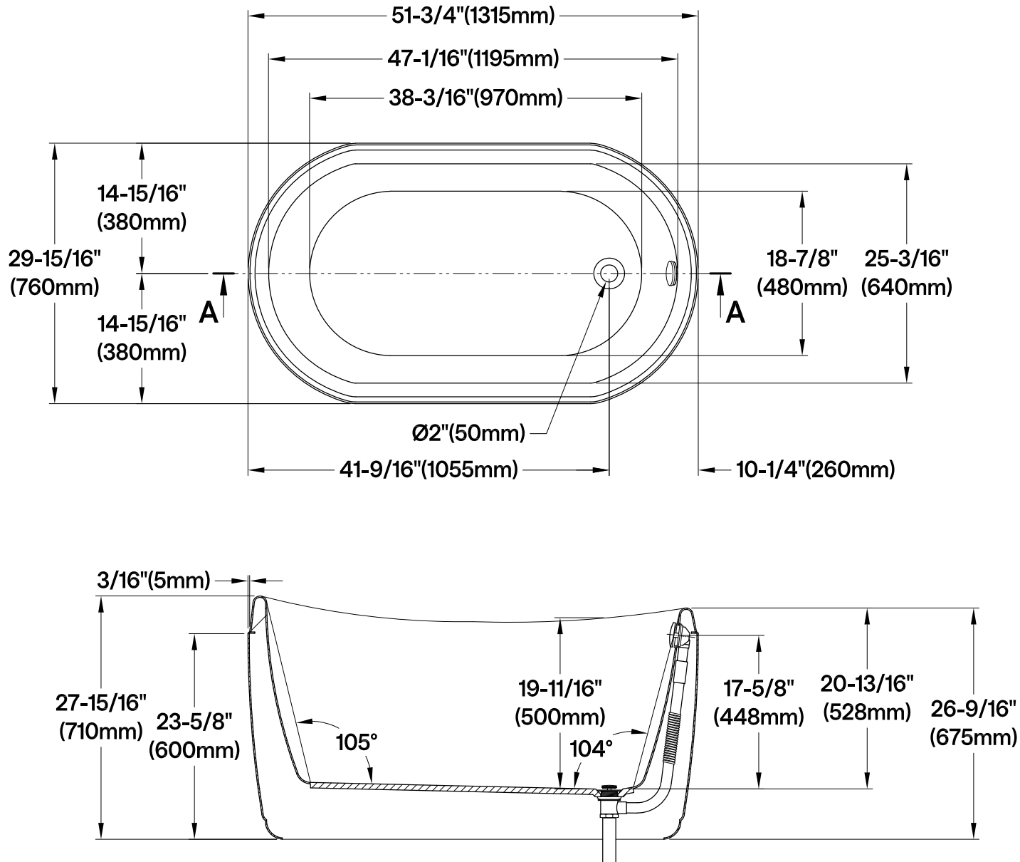
Section A-A
