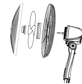
1. Assemble Fan Head
