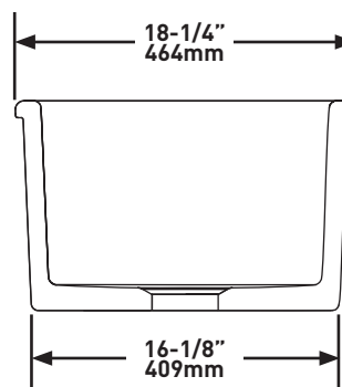
Vista frontal de la sección transversal
