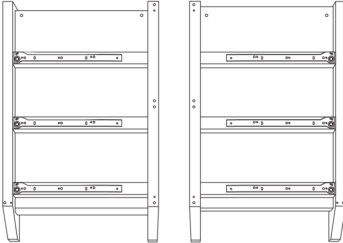
A. Left Side Panel A. Panneau latéral gauche B. Right Side Panel B. Panneau latéral droit
