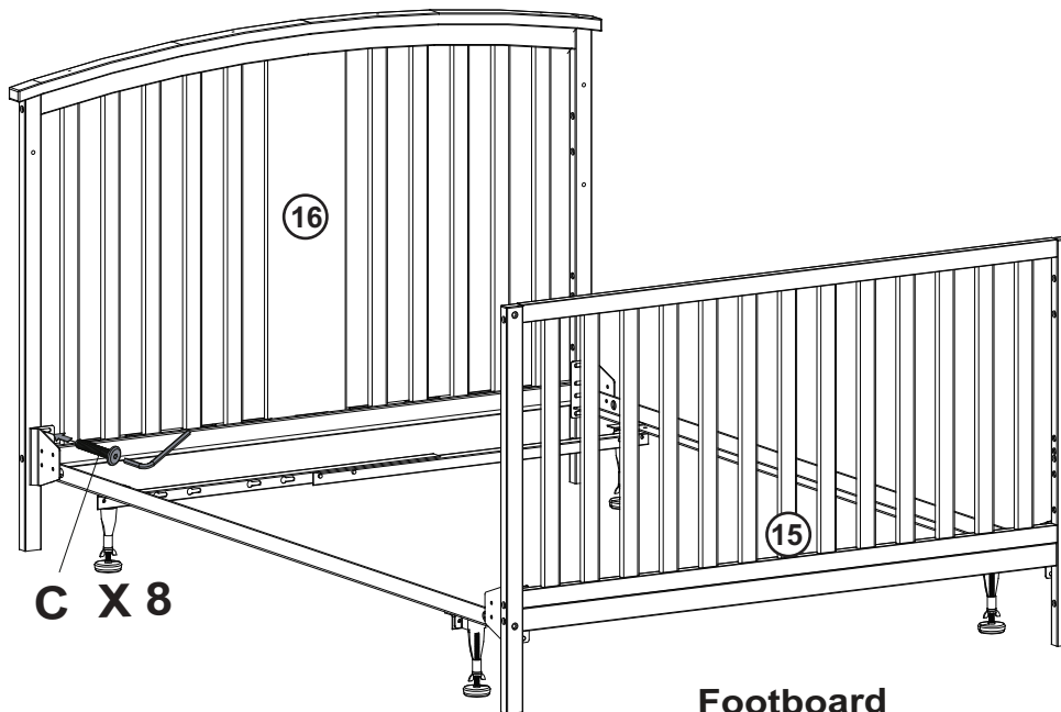
Headboard tête de lit cabecera
