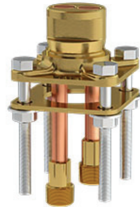
Válvula de llenador de bañera para montaje en suelo
